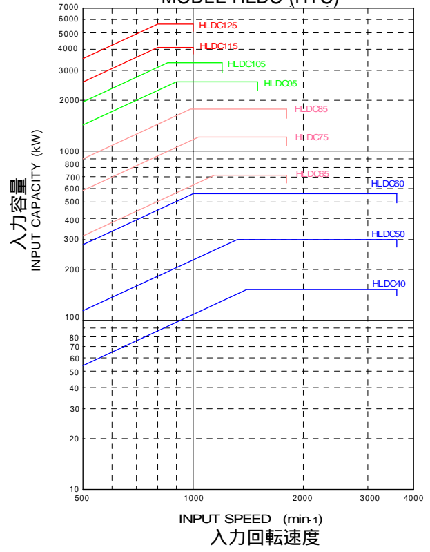
ファン・ブローア用 CAPACITY CHART OMEGA CLUTCH FOR FAN, BLOWER MODEL HLDC (HYC)
