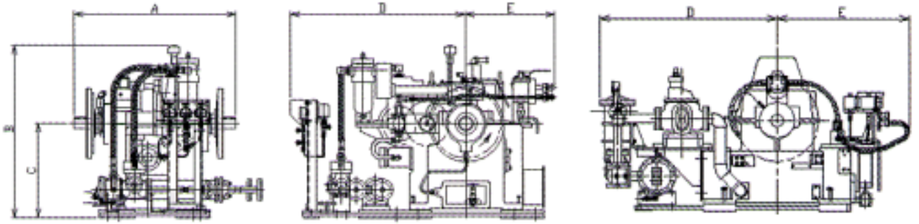
HY(C)65 ~ 125形(電動潤滑油ポンプ付)
